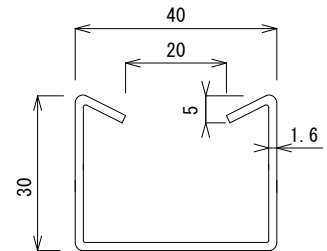
レール断面詳細図 溶融垂鉛メッキ仕上
