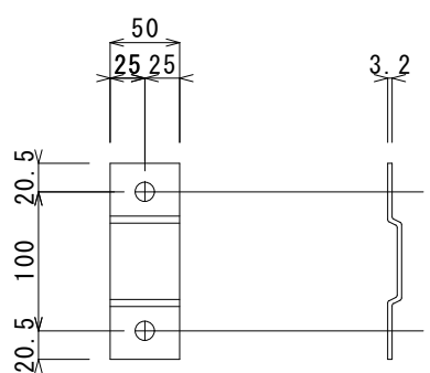
連結金具 詳細図
