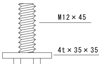
取付ボルトA 詳細図
