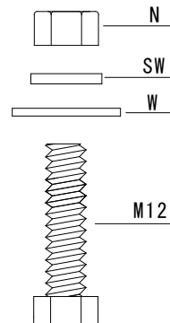
取付ボルトA 詳細図
