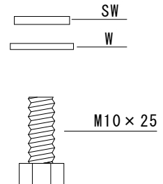
取付ボルトB 詳細図
