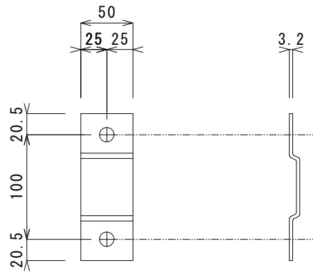
連結金具 詳細図
