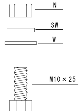
取付ボルトB 詳細図
