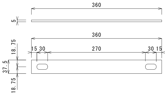
連結金具 詳細図
