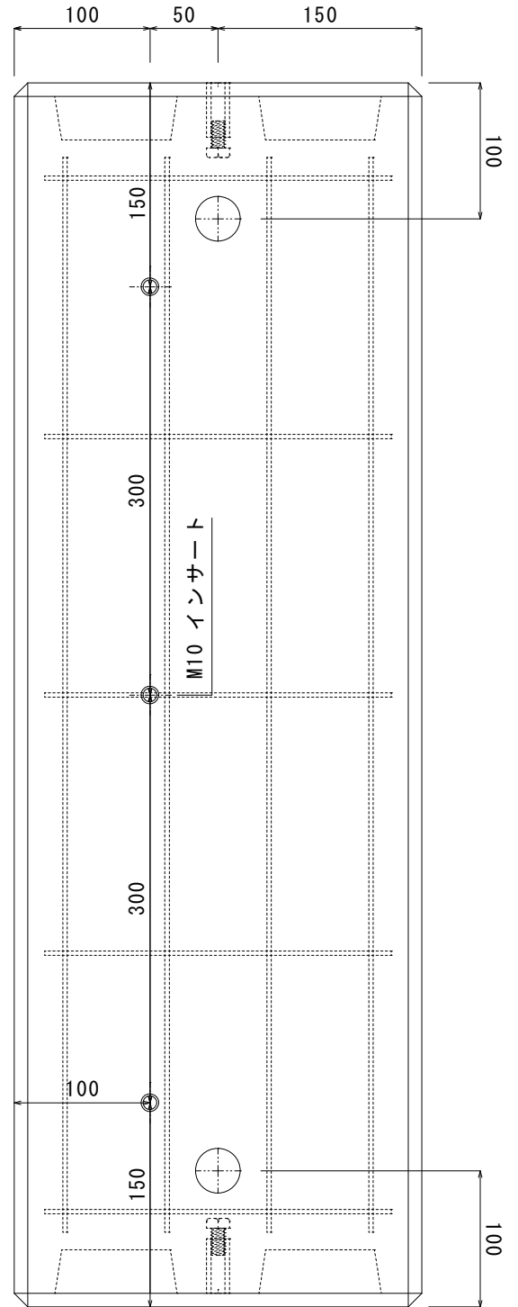
《平面図》
