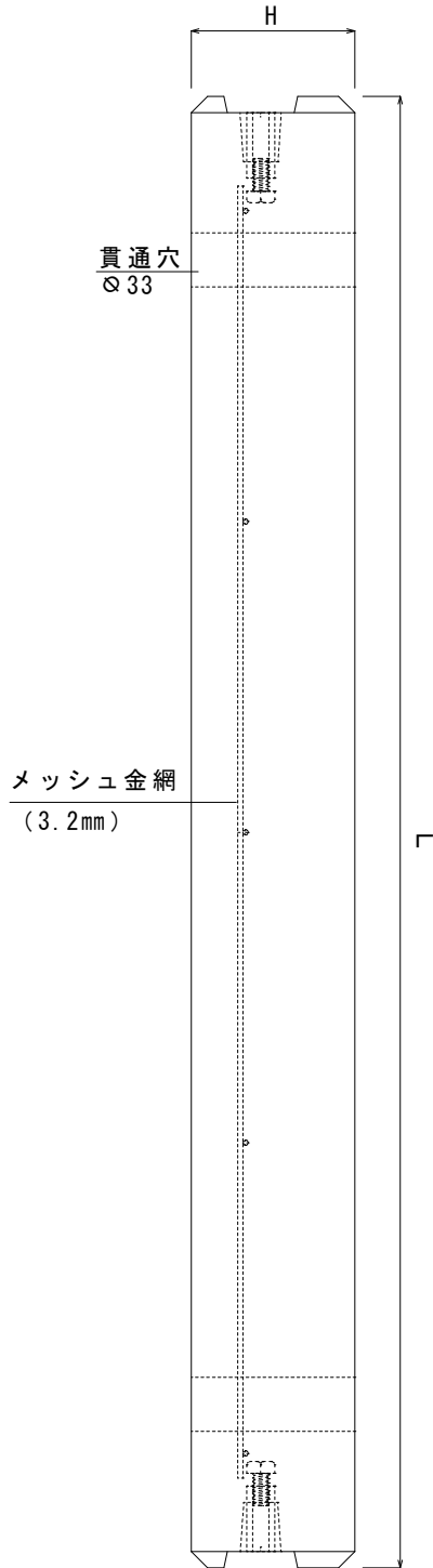
《側面図》
