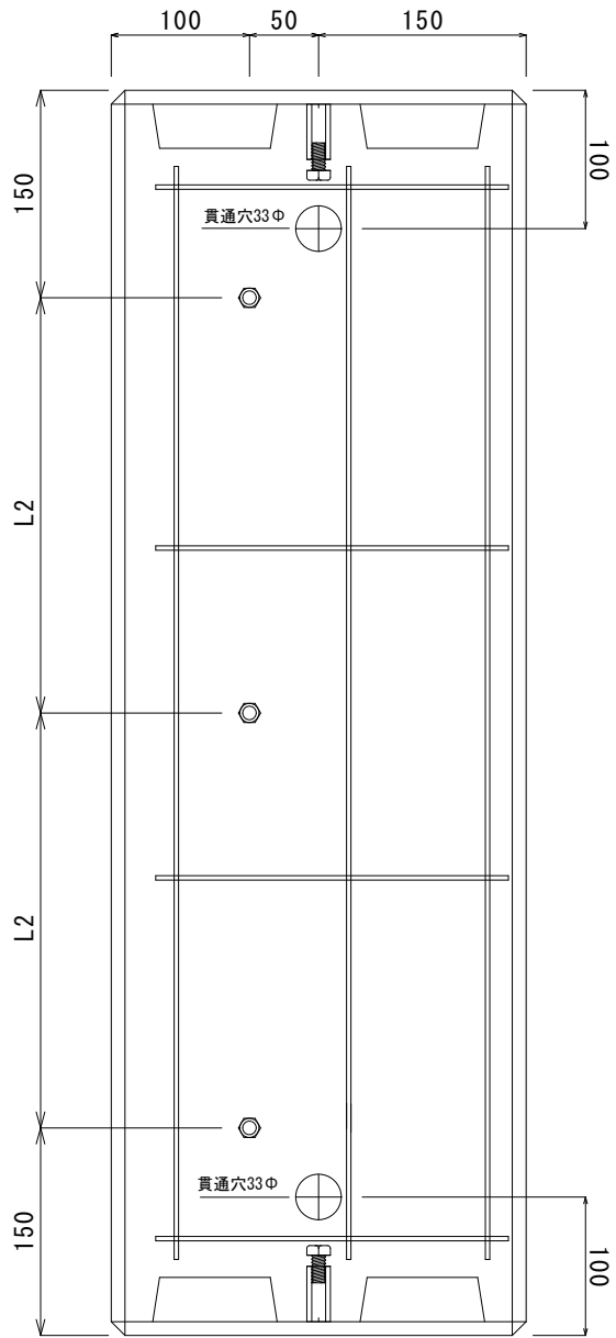
《断面図》
