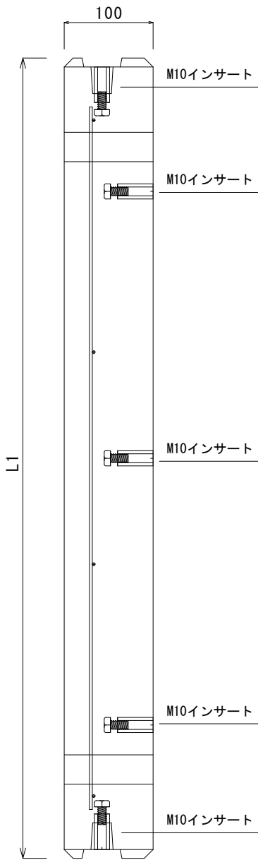
《側面図》
