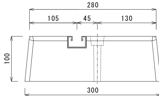
《断面図》
