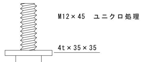
取付ボルト詳細図
