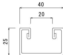
レール部詳細図
