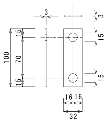
連結金具 詳細図
