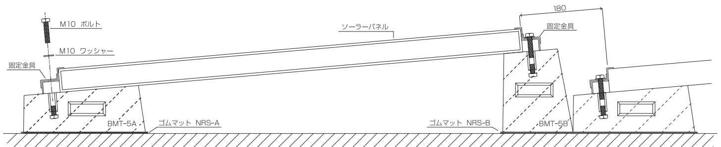
施工例1 (イメージ)
