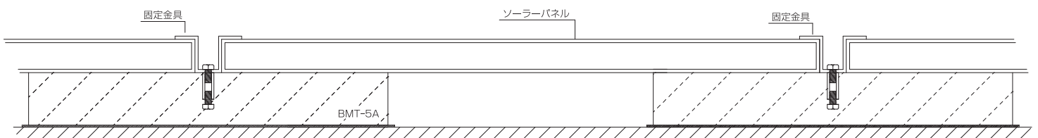
施工例2 (イメージ)
