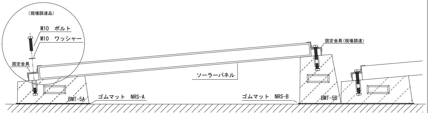
施工例 1 (イメージ)
