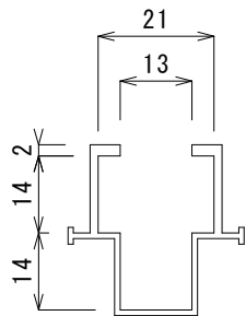
アルミレール断面詳細図 アルミアルマイトクリア加工 W1/2 対応
