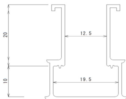
新型のM12アルミレール
