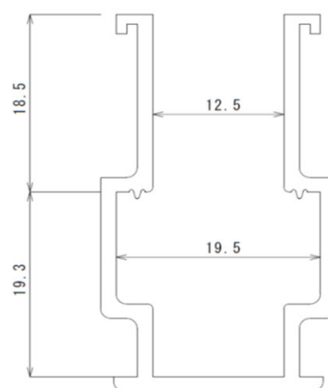
従来のM12アルミレール
