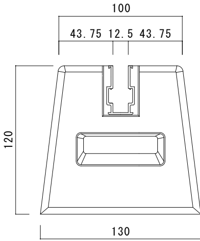
断面図
