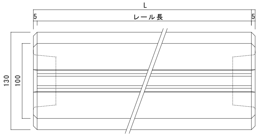
平面図
