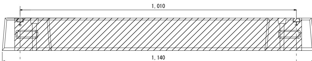
アルミレール外側設置 最大アンカーピッチ
