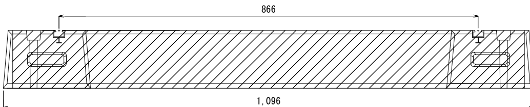
アルミレール内側設置 最小アンカーピッチ
