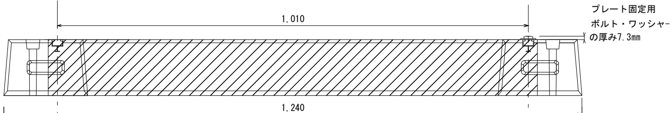
アルミレール内側設置 最大アンカーピッチ
