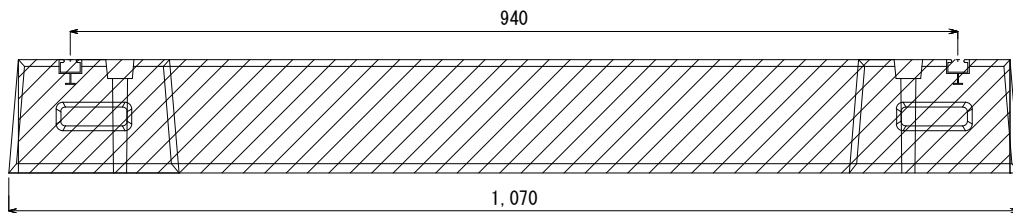
アルミレール外側設置 最小アンカーピッチ
