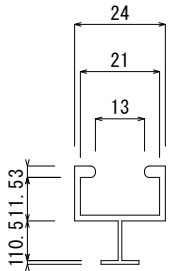
4分アルミレール詳細図
